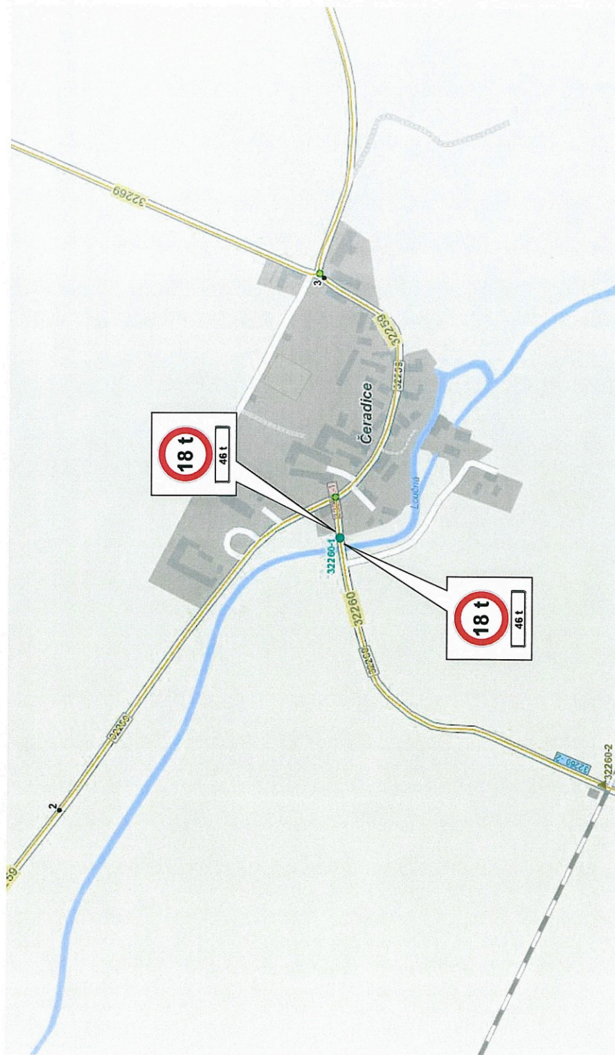
Příloha č. 1: Grafický návrh osazení přechodného SDZ, mostní objekt ev. č.: 32260 – 1
